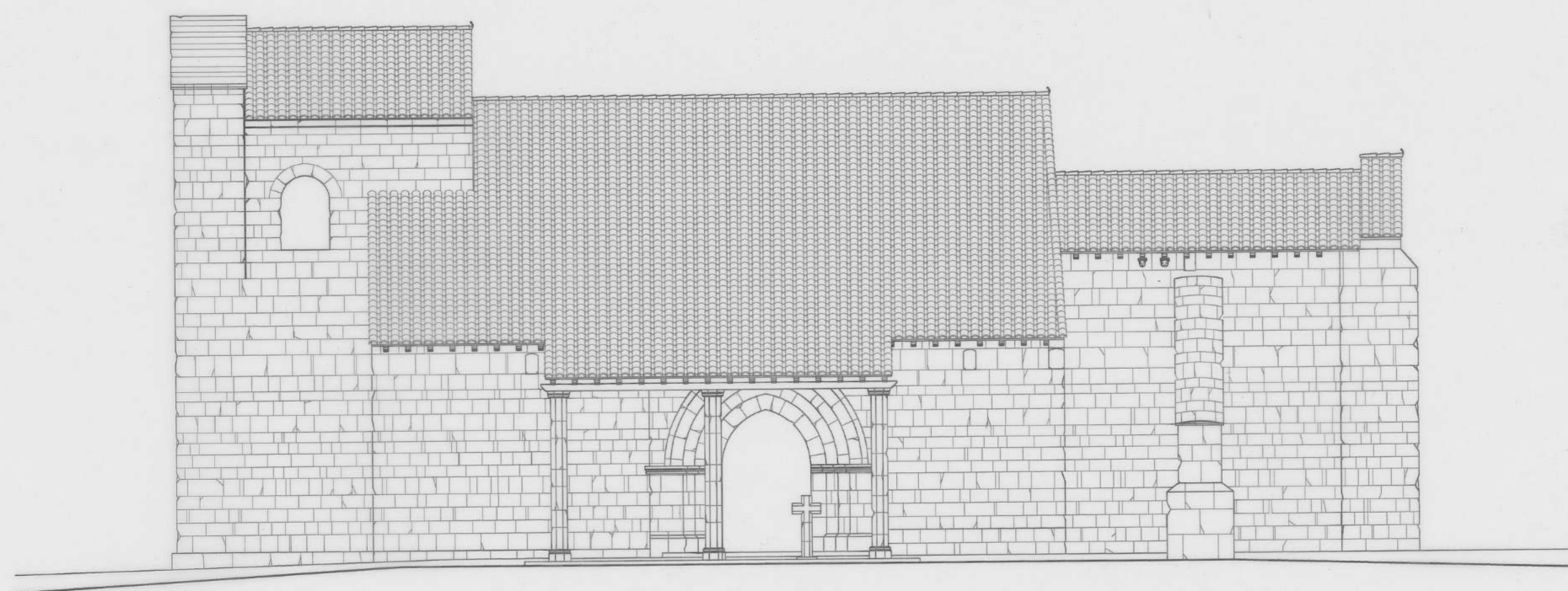
ALZADO SUR
