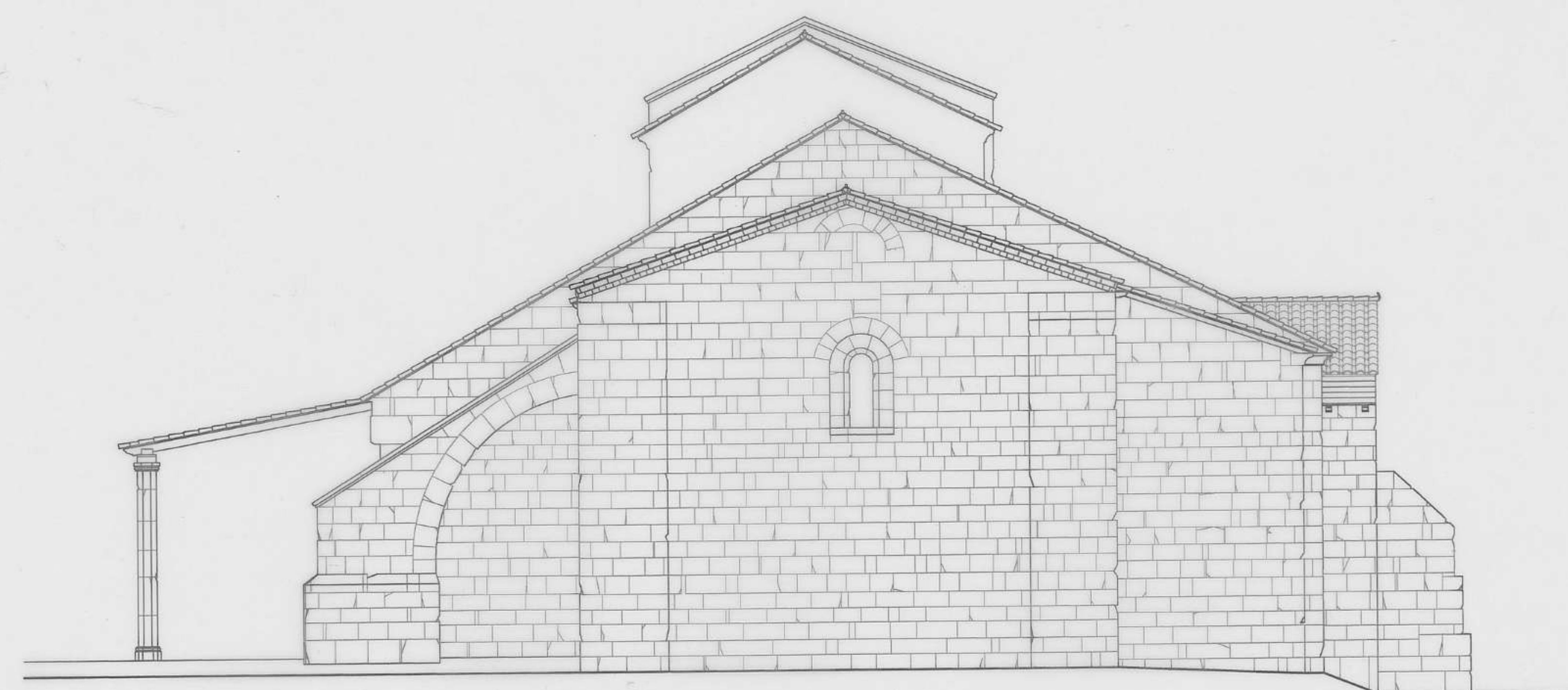
ALZADO ESTE
